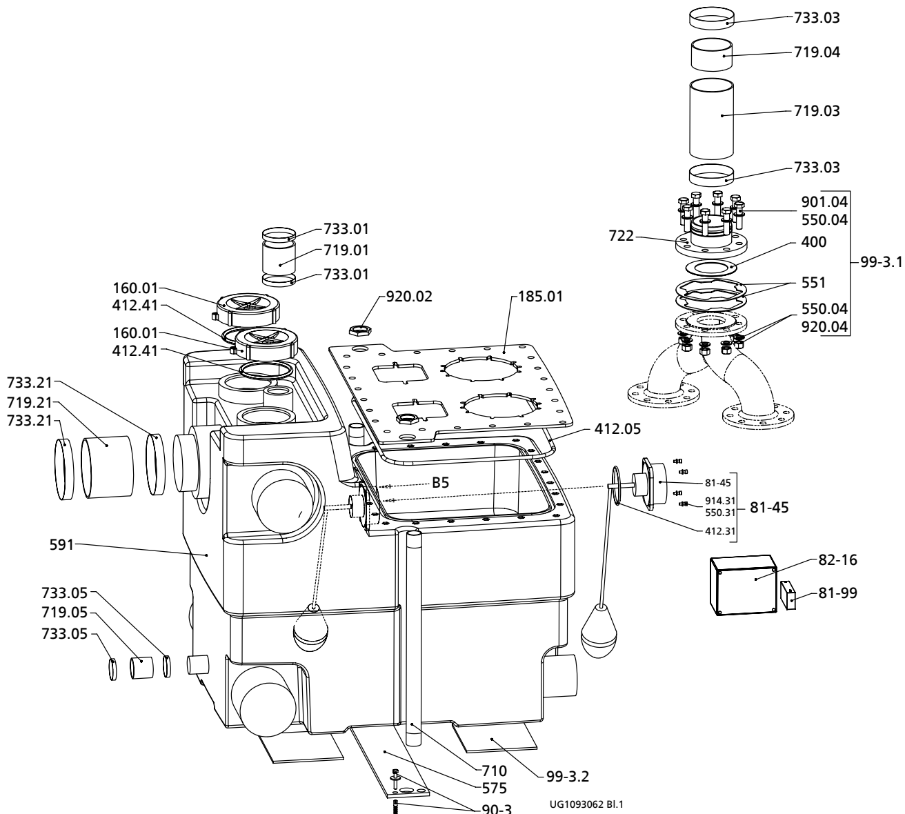
Рис. 32: Покомпонентный сборочный чертеж Compacta UZ450 и UZ900
