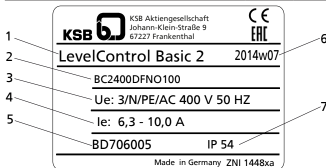
Рис. 2: Заводская табличка
