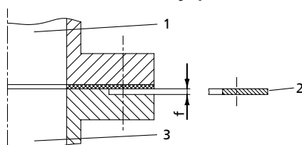
Рис. 9: Фланцевое соединение
