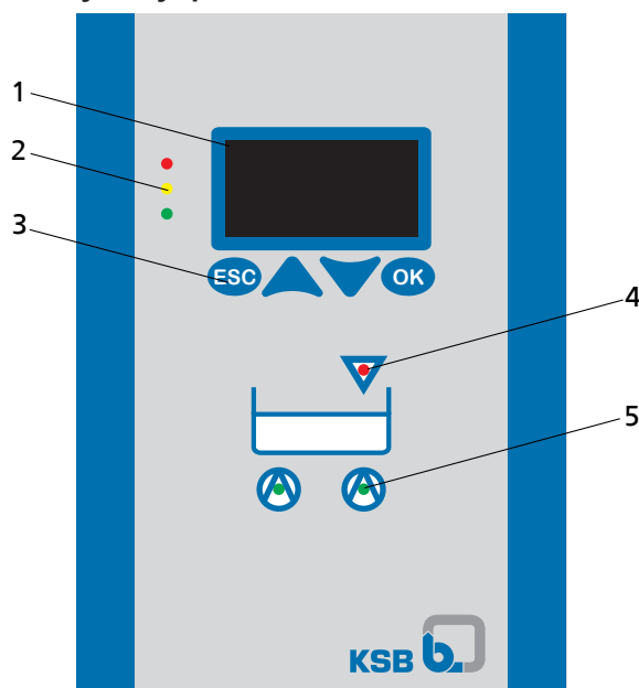
Рис. 21: Панель управления
