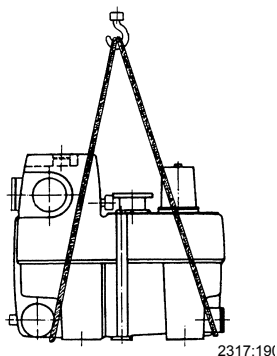
Рис. 1: Транспортировка резервуара для Compacta UZ450 и UZ900
