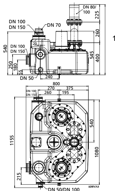
Рис. 38: Габариты Compacta UZ150, UZ300
