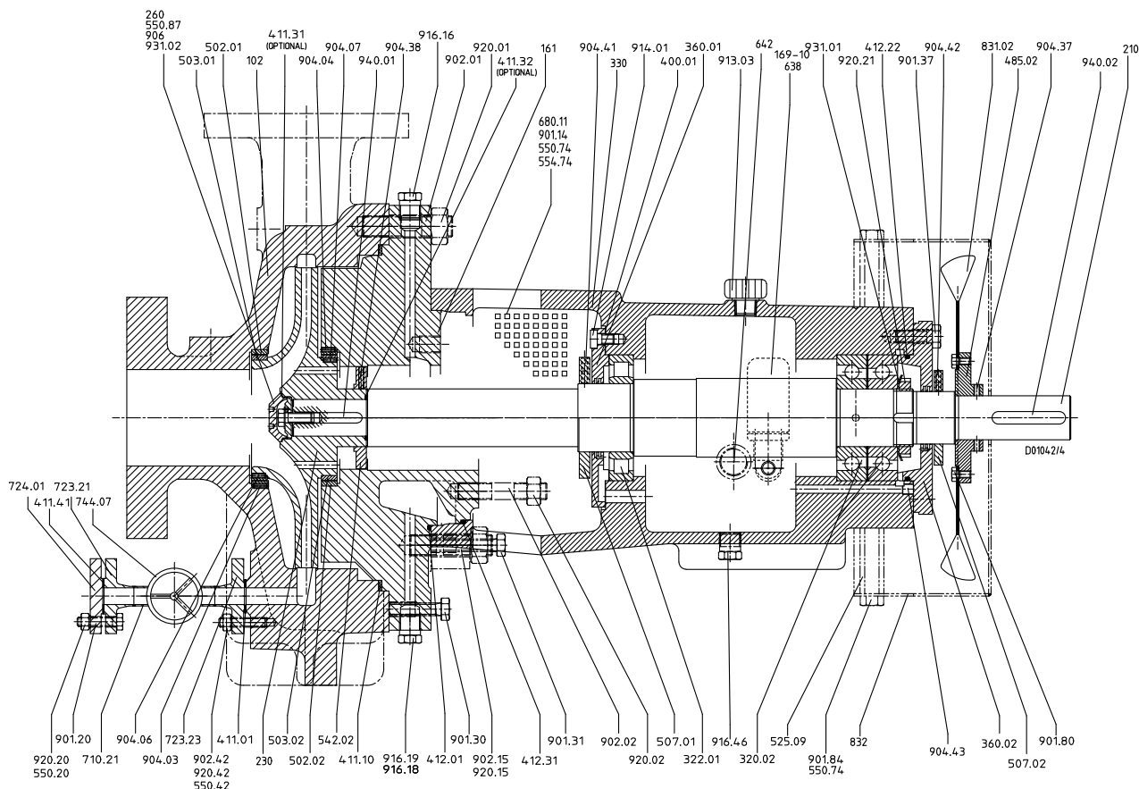
Рис. 15: Корпус подшипника B02–B05, а) без охлаждения и б) с охлаждением
