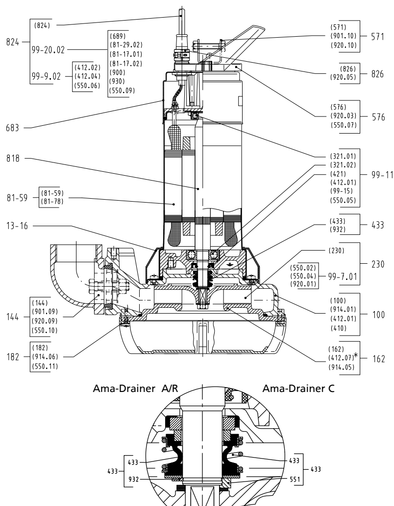
Рис. 7: Сборочный чертеж Ama-Drainer 522/11
