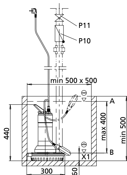
Рис. 8: Чертеж с размерами Ama-Drainer 4..SE/10 без рубашки охлаждения
