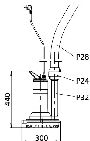
Рис. 12: Чертеж с размерами Ama-Drainer 4..NE/10 без рубашки охлаждения
