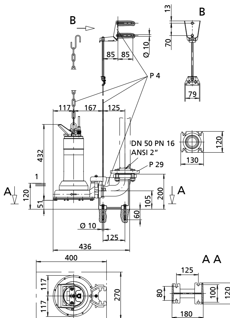
Рис. 16: Чертеж с размерами Ama-Drainer 522 ND/11 с направляющим тросом
