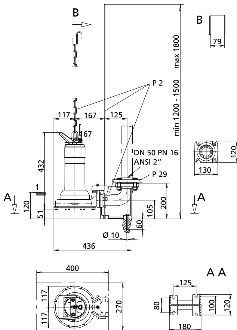
Рис. 15: Чертеж с размерами Ama-Drainer 522 ND/11 со скобой
