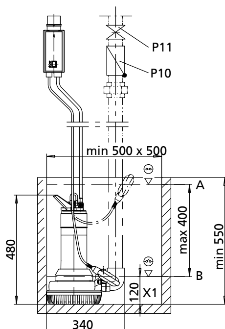
Рис. 11: Чертеж с размерами Ama-Drainer 522/11 без рубашки охлаждения
