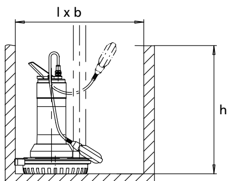
Рис. 3: Установка — размеры
