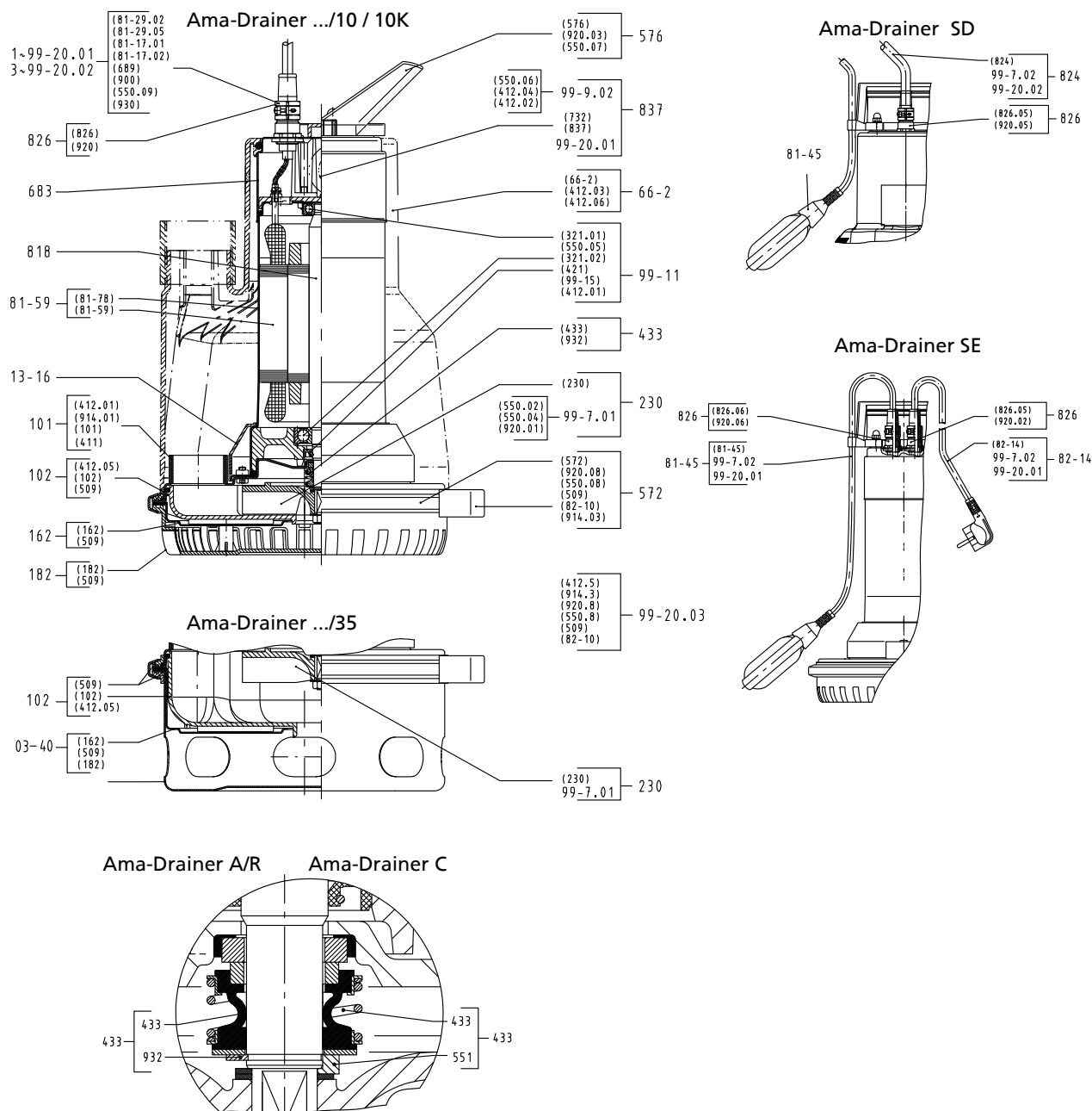
Рис. 6: Сборочный чертеж Ama-Drainer .../10, .../10K, .../35
