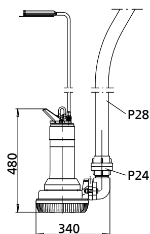
Рис. 14: Чертеж с размерами Ama-Drainer 522 ND/11 без рубашки охлаждения
