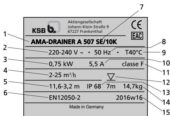
Рис. 1: Заводская табличка (пример)
