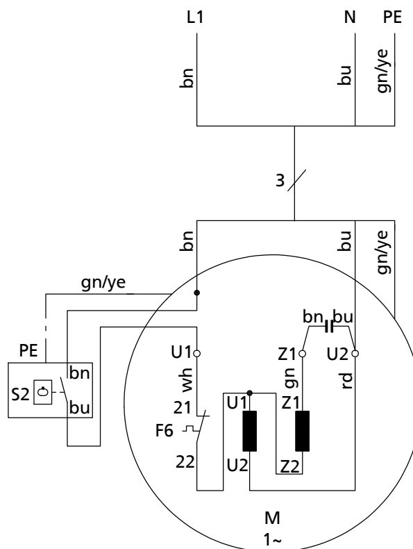
Рис. 18: Электрическая схема подключения Ama-Drainer SE
