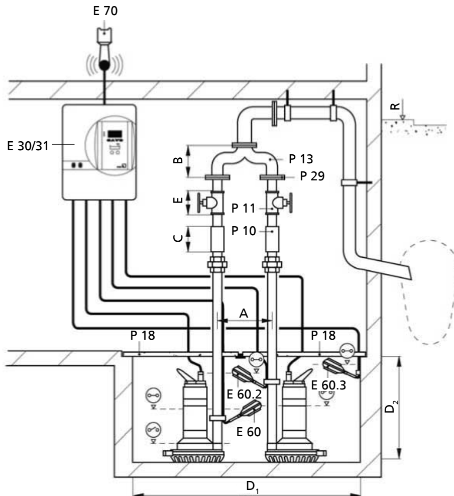
Рис. 17: Расположение поплавковых выключателей в двойной насосной установке
