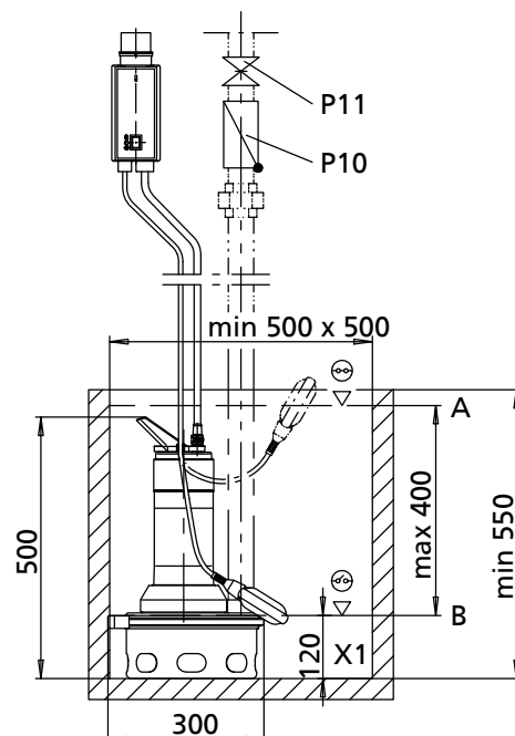
Рис. 10: Чертеж с размерами Ama-Drainer 4..SD/35 без рубашки охлаждения
