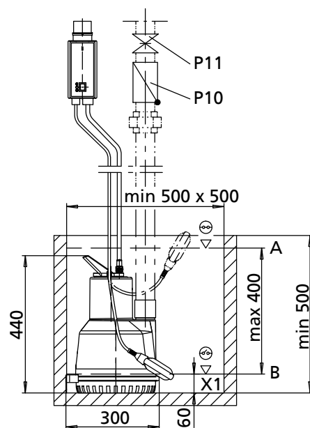
Рис. 9: Чертеж с размерами Ama-Drainer 5..SD/10 K с рубашкой охлаждения
