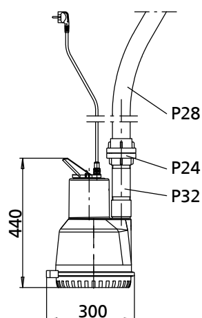
Рис. 13: Чертеж с размерами Ama-Drainer 5..NE/10 K с рубашкой охлаждения
