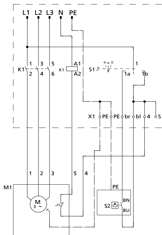
Рис. 20: Электрическая схема подключения Ama-Drainer SD
