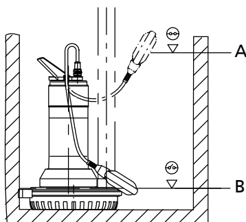
Рис. 4: Точка включения/выключения
