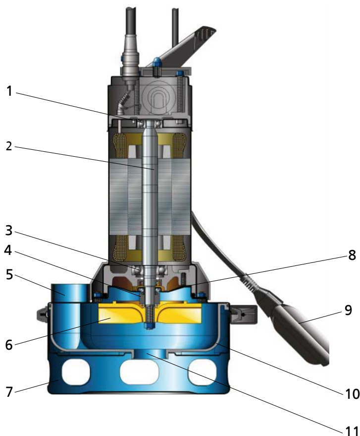
Рис. 2: сечение
