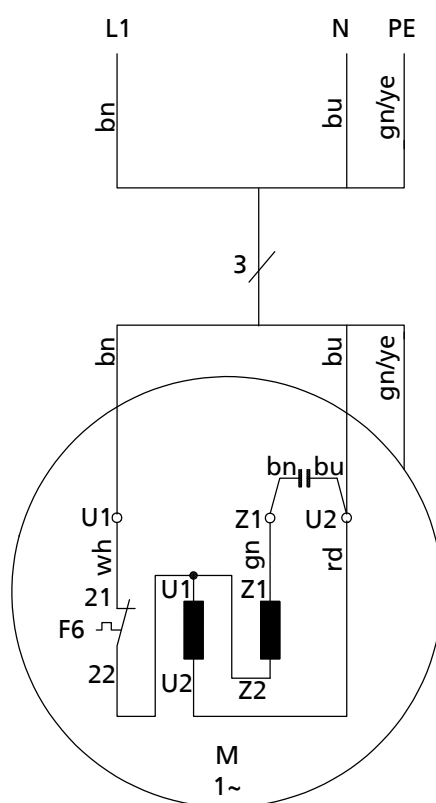
Рис. 19: Электрическая схема подключения Ama-Drainer NE
