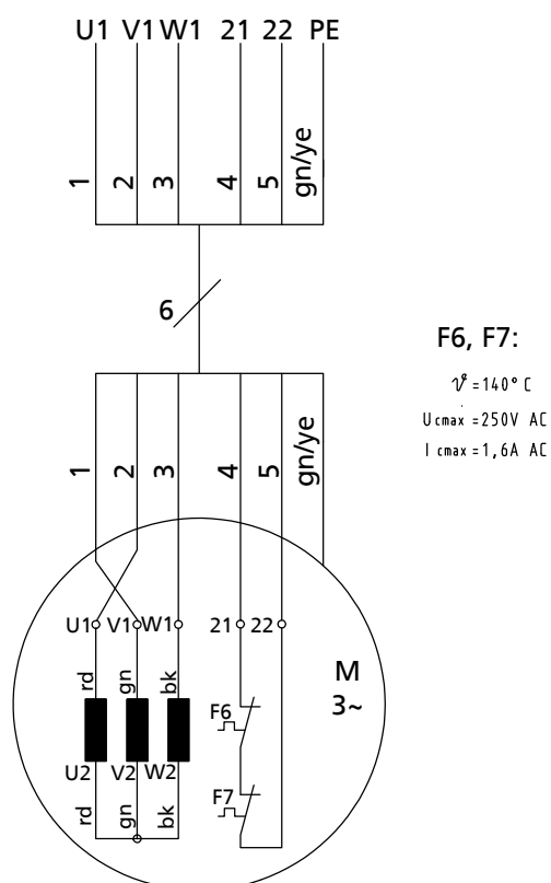
Рис. 21: Электрическая схема подключения Ama-Drainer ND
